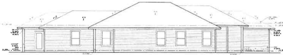
4 A3 ELEVATION A LEFT ELEVATION SCALE: 3/32" = 1'-0"
