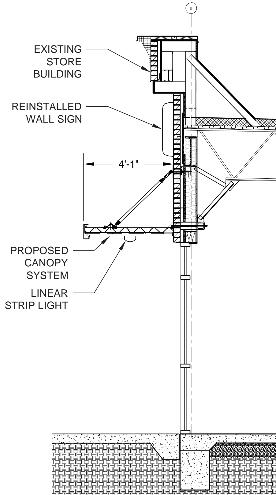
SECTION A-A
