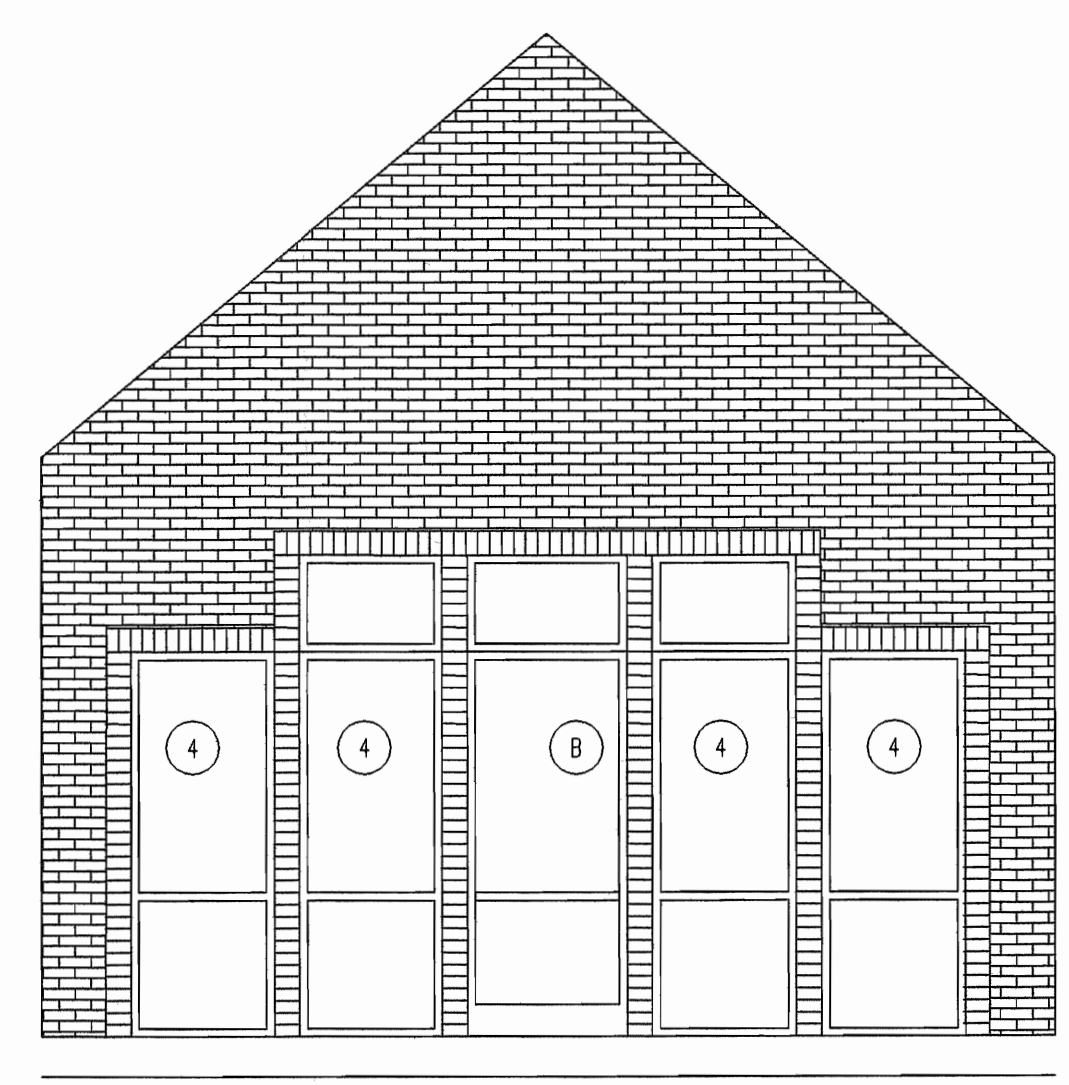
04 PORCH ELEVATION SCALE: 1/4" = 1'-0"
