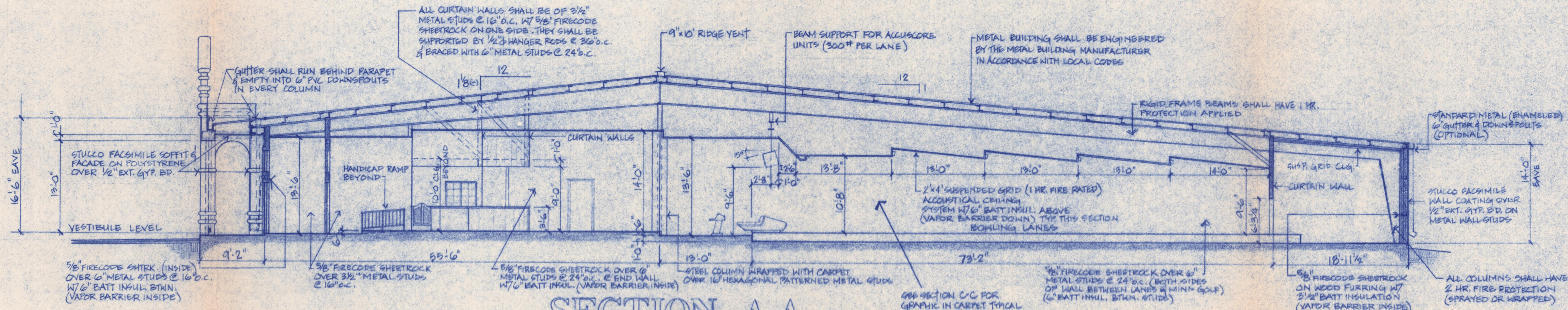
SECTION A-A 1/8" = 1'-0"
