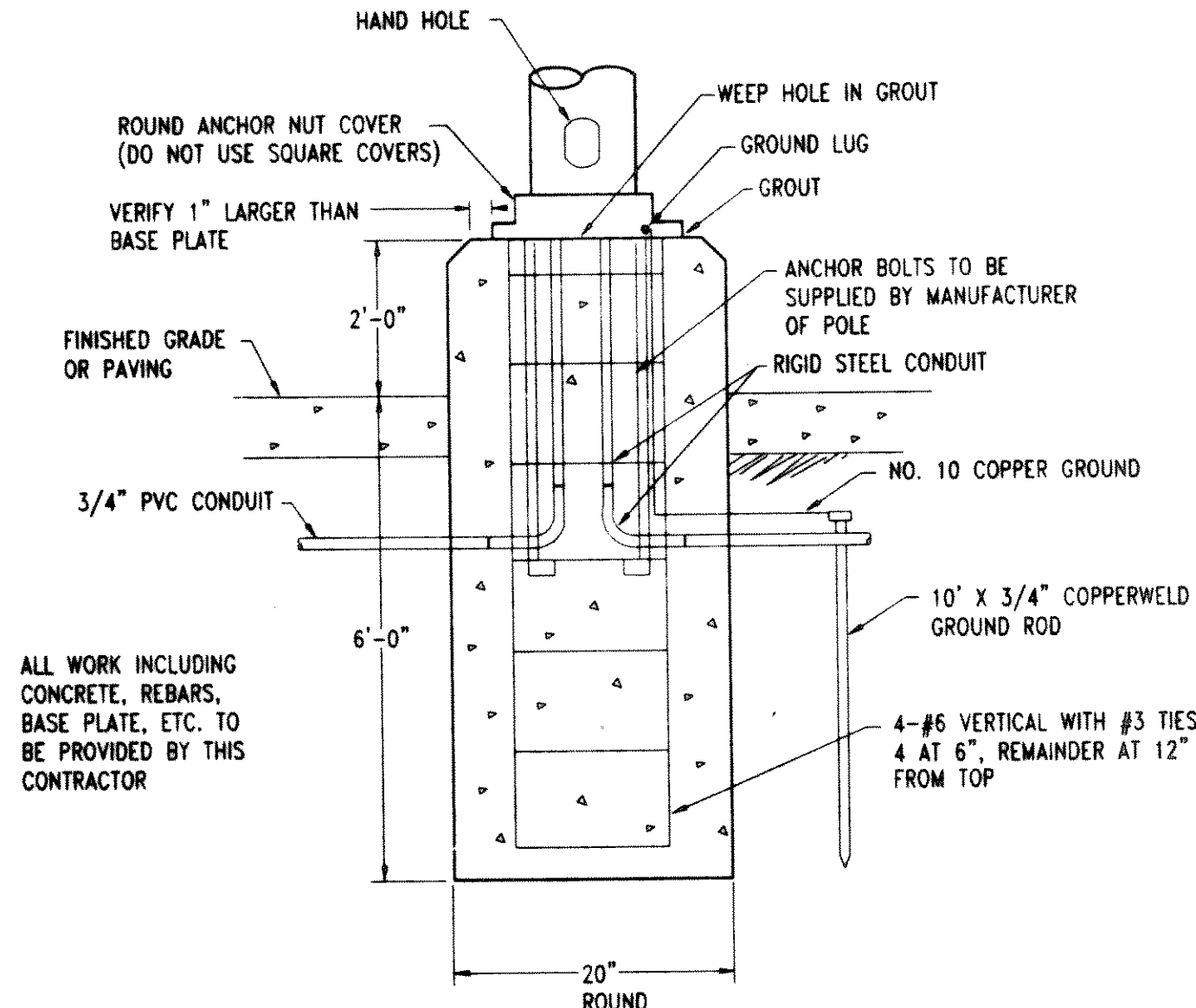
2 POLEBASE DETAIL 9.0 N.T.S.
