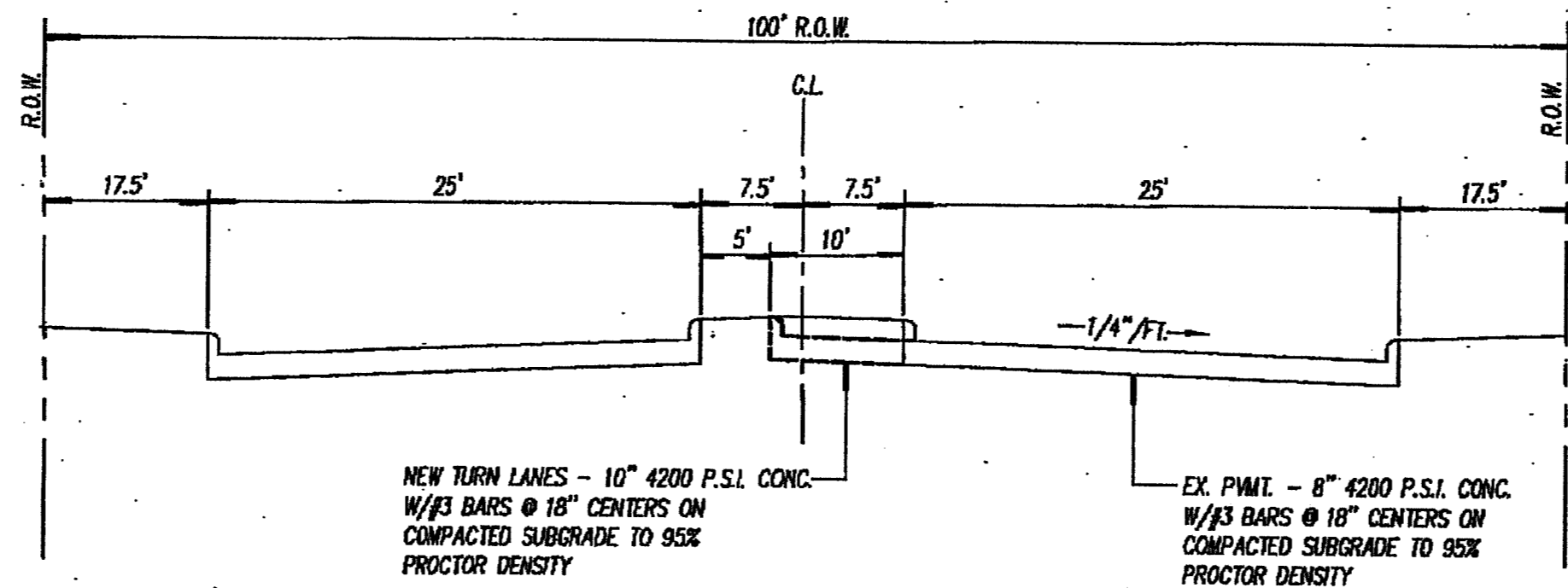
PROP. PAVEMENT DETAIL N.T.S.
