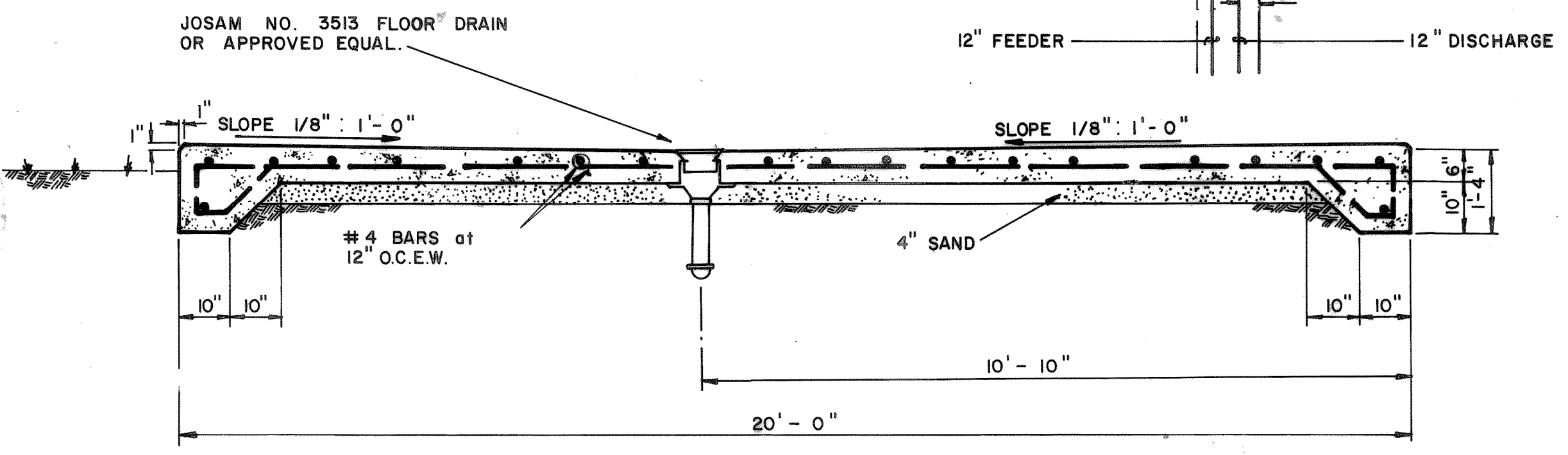
SECTION 2 SCALE: 1/2" = 1'-0"
